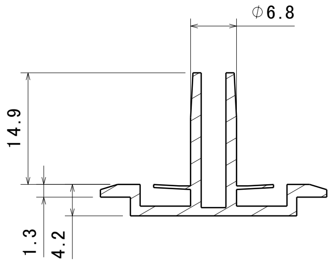
截面分割 A-A 缩放: 2:1
